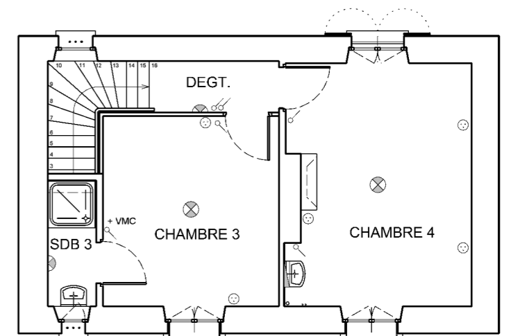
PLAN DE NIVEAU 1 - ECH. 1.100 ème
