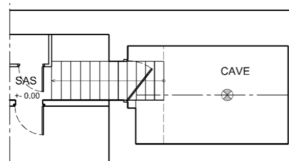
PLAN DE LA CAVE - ECH. 1.100 ème
