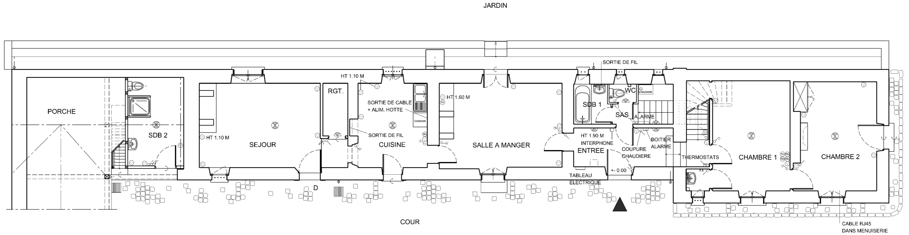
PLAN DE REZ DE CHAUSSEE - ECH. 1.100 ème
